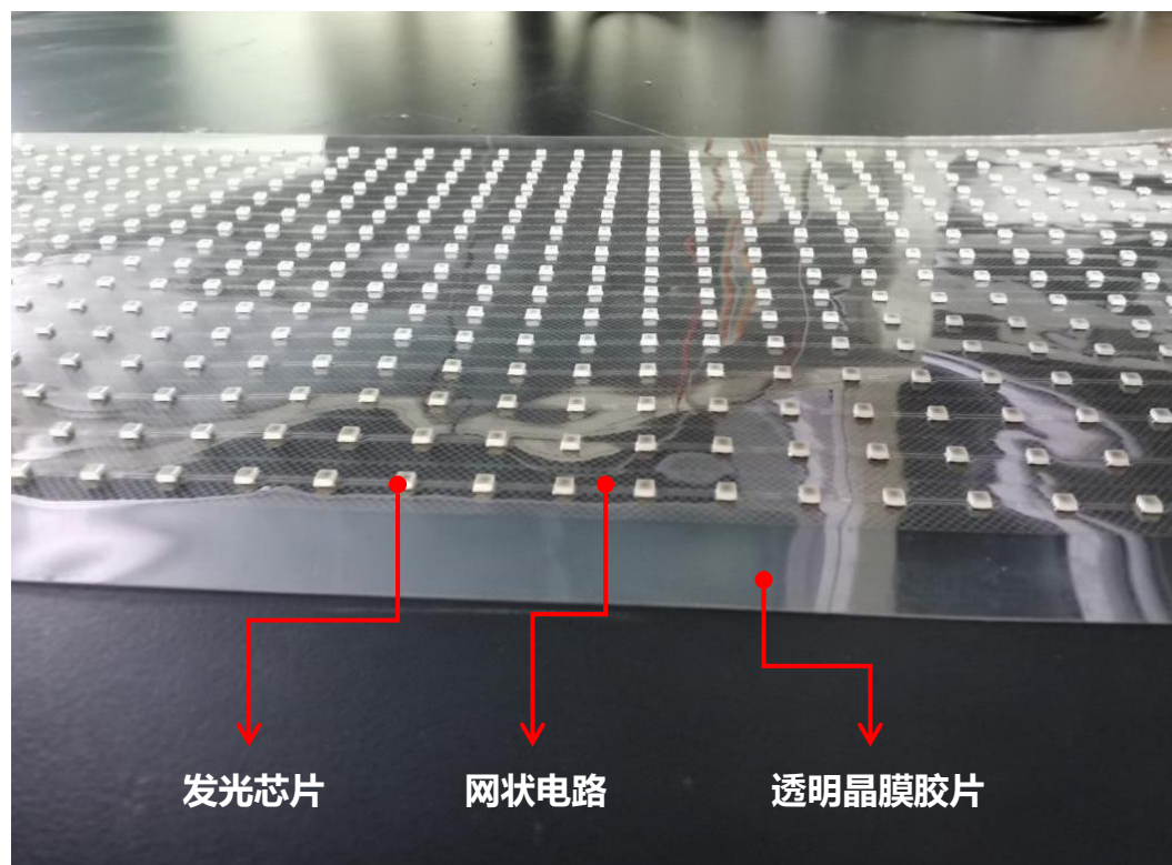
产品结构示意
